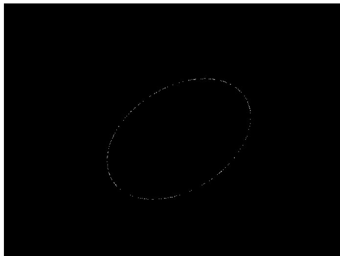
Figure 5.10.2: glm::vec4(glm::circularRand(1.0f), 0, 1);
