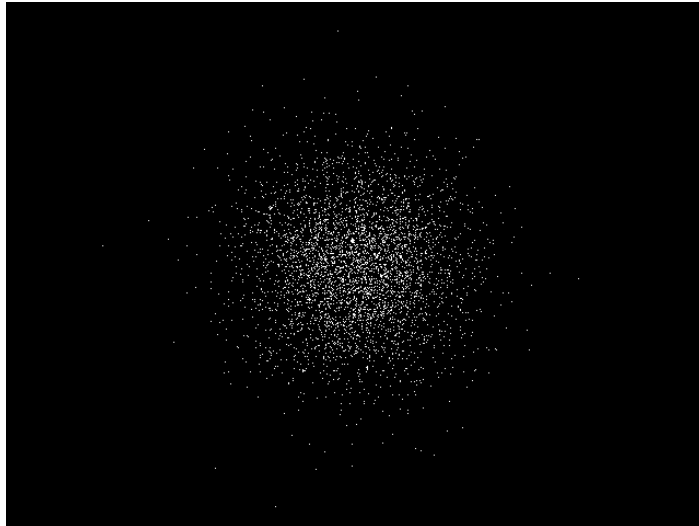
Figure 5.7.6: glm::vec4(glm::gaussRand(glm::vec3(0), glm::vec3(1)), 1);
