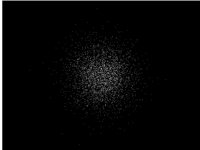
Figure 5.10.6: glm::vec4(glm::gaussRand(glm::vec3(0), glm::vec3(1)), 1);
