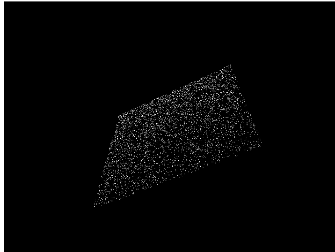
Figure 5.10.1: glm::vec4(glm::linearRand(glm::vec2(-1), glm::vec2(1)), 0, 1);
