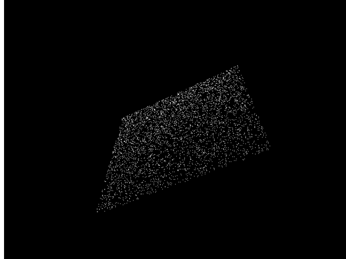
Figure 4.8.1: glm::vec4(glm::linearRand(glm::vec2(-1), glm::vec2(1)), 0, 1);
